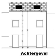
Achtergevel
