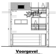
Voorgevel
